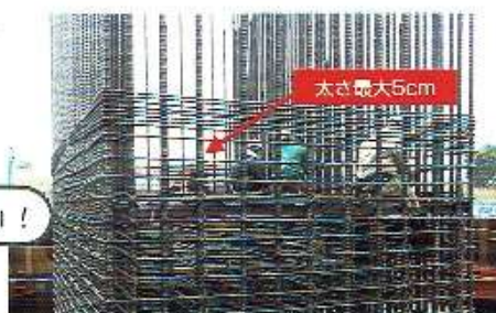
コンクリート橋脚の鉄筋
